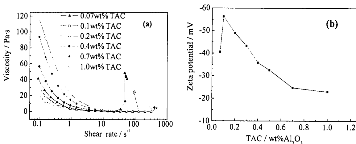
图 1 不同 TAC 加入比例对 55vol% 氧化铝悬浮液流变特性 (a) 及 Zeta 电位 (b) 的影响
