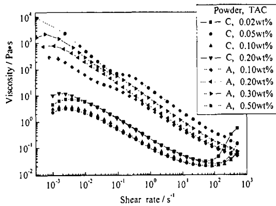
图 3 不同粒度氧化铝 50vol% 悬浮液的流变曲线
