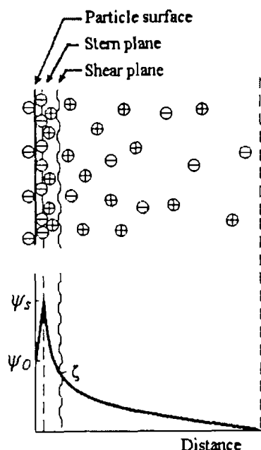
图 2 柠檬酸铵稳定的氧化铝悬浮液中颗粒表面的双电层结构和相应电势示意图
